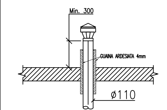
PARTICOLARE TIPICO ESALAZIONE COLONNA DI SCARICO
